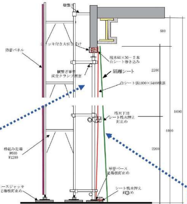
図 4.7.16 外壁の飛散防止措置模式図（開口部を防火シートで塞ぎ頭部と脚部及び高さに応じて中間部を固定）
