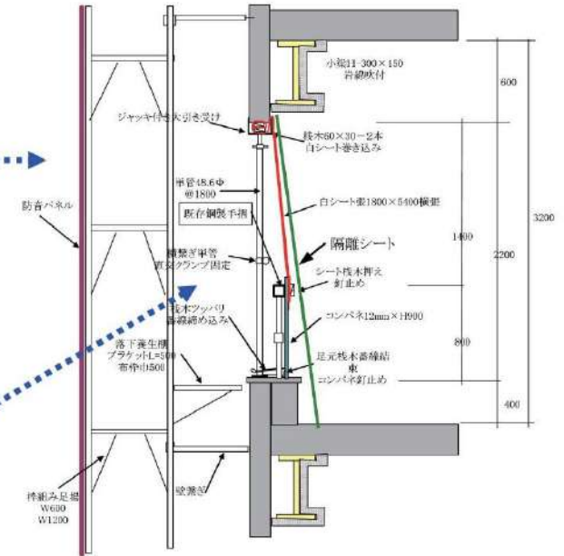
図 4.7.15 外壁の飛散防止措置模式図（開口部を防火シートで塞ぎ、手すりにベニヤ板を張ったシートの内部側に隔離用プラスチックシート等を張る）
